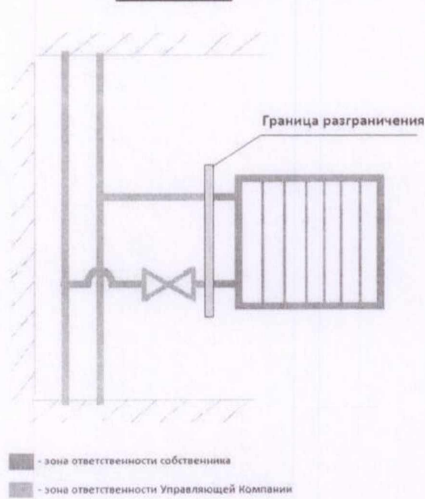
Граница разграничения ответственности по отоплению
